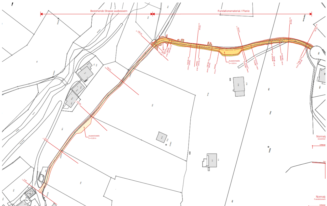
Plan 4: Situaziun sviament provisorii
