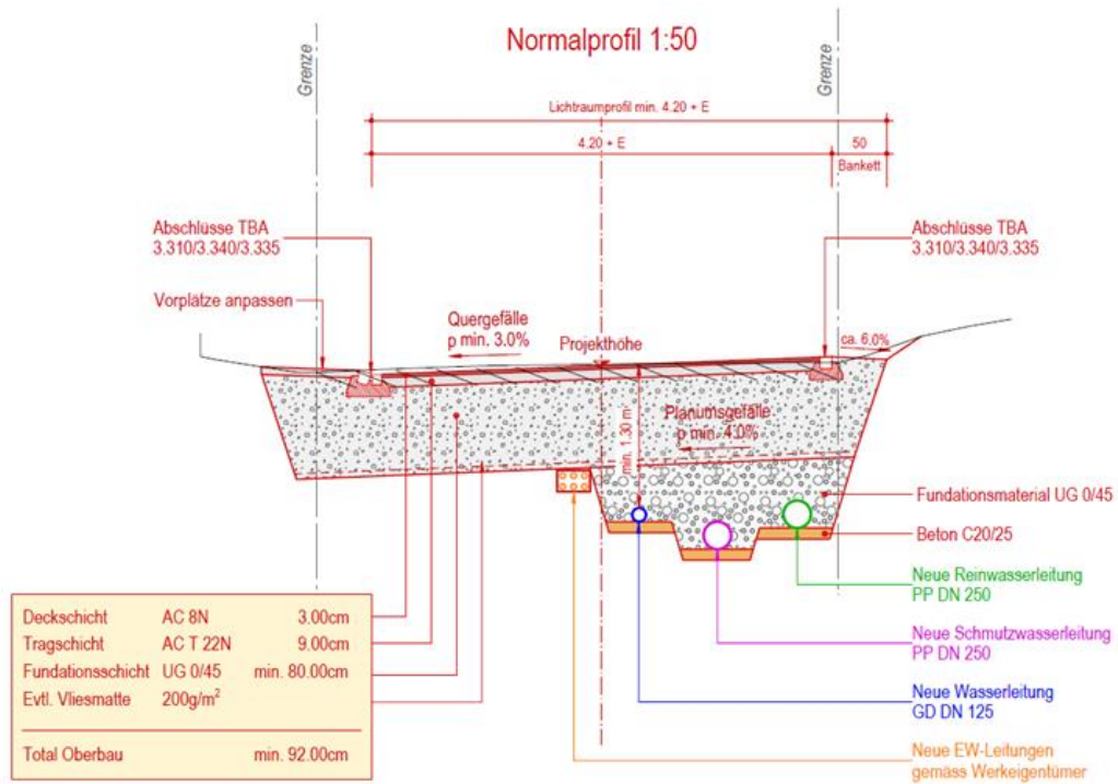
Plan 3: Profil normal via
